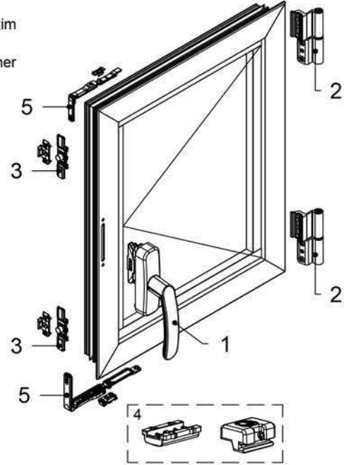
4 - 0710621 Kanat Kaldırma Takoğu, bütün açılır Pencere kanatları altında 1 adet kullanılır.
