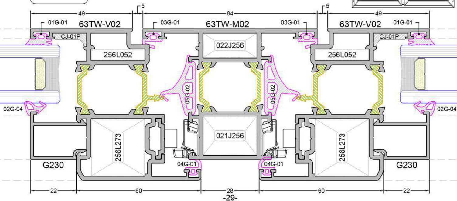
DETAY - 2a DETAIL - 2a
